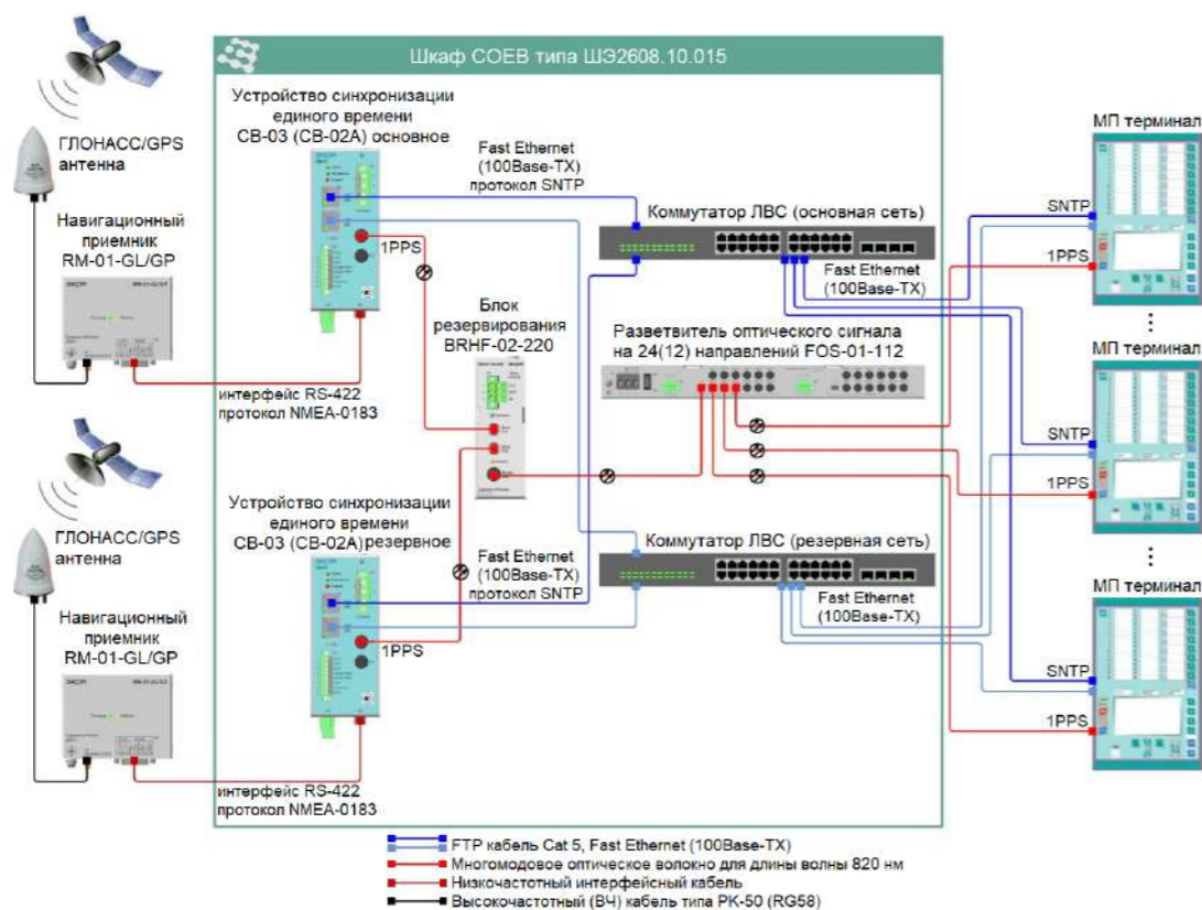
СТРУКТУРНАЯ СХЕМА ШКАФА С УСТРОЙСТВОМ СИНХРОНИЗАЦИИ ЕДИНОГО ВРЕМЕНИ СВ-03 (СВ-02А)
