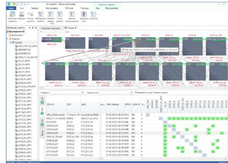
Привязки GOOSE-сообщений
