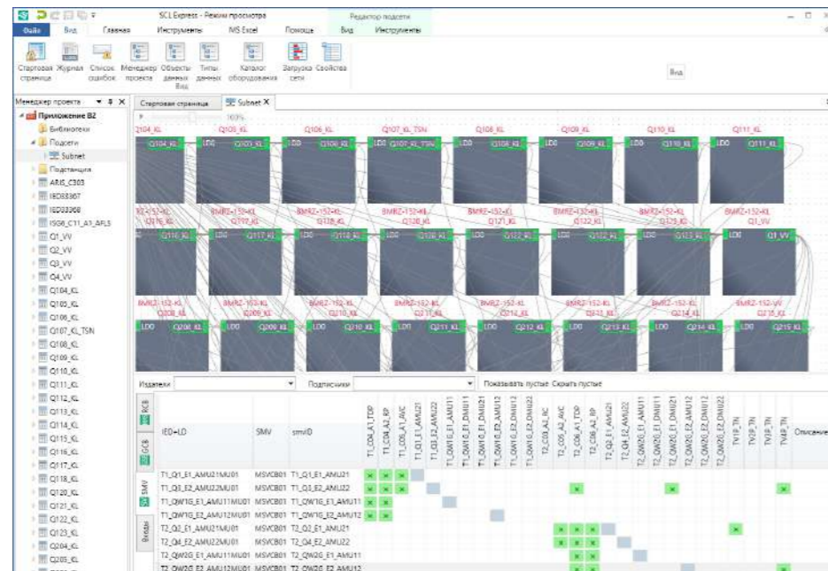
Привязки SV-сообщений
